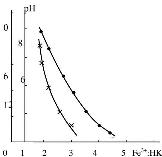
Рисунок 2. Зависимость уменьшения общей щелочности воды и pH от соотношения Fe^{3+}:HK в системе: V_o:V_b=0,008 ● – щелочность, × – pH раствора
