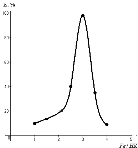
Рисунок 1. Зависимость извлечения нефтяных кислот от соотношения Fe^{3+}:HK в системе
